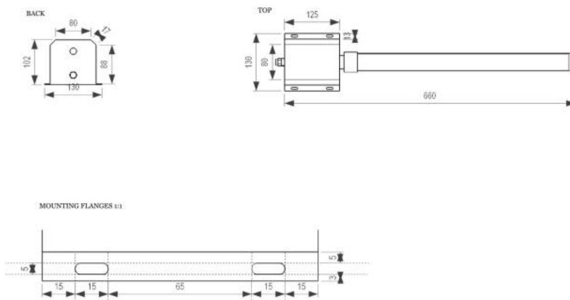
Kuva 1. Laitteen mitat (mm).
